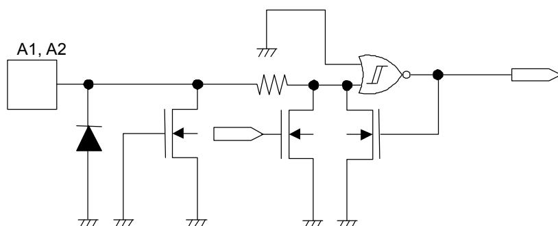
図22 A1, A2端子
