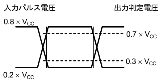
図3 AC測定入出力波形
