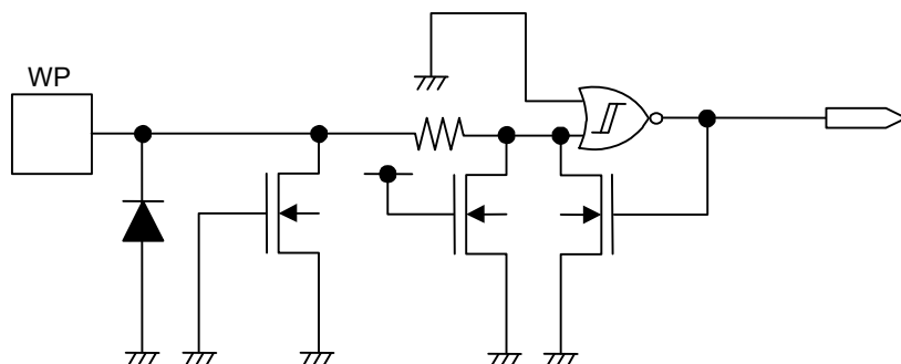
図21 WP端子
