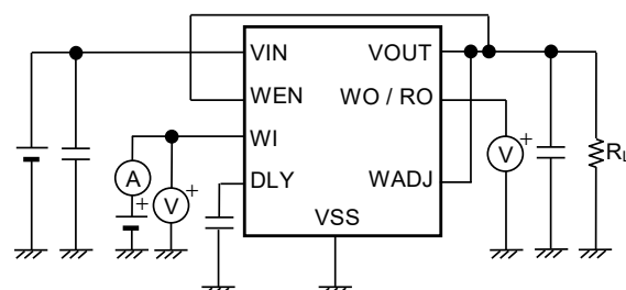
図19 測定回路8
