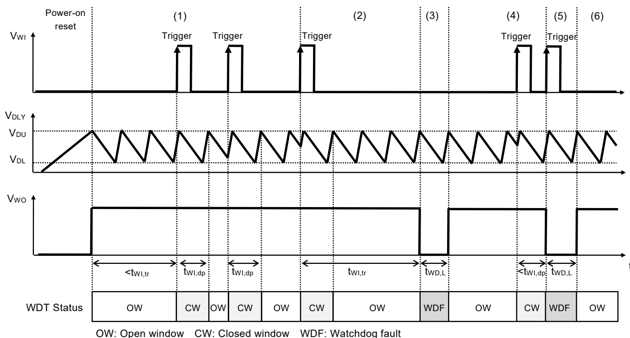
図37 ウォッチドッグタイマ部のタイミングチャート
