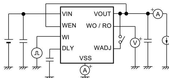
図21 測定回路10
