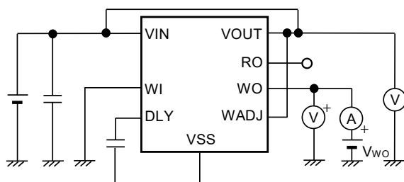
図30 測定回路9
