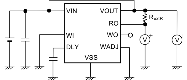
図25 測定回路4
