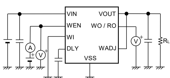
図20 測定回路9
