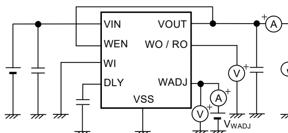
図18 測定回路7
