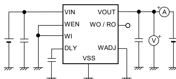
図13 測定回路2
