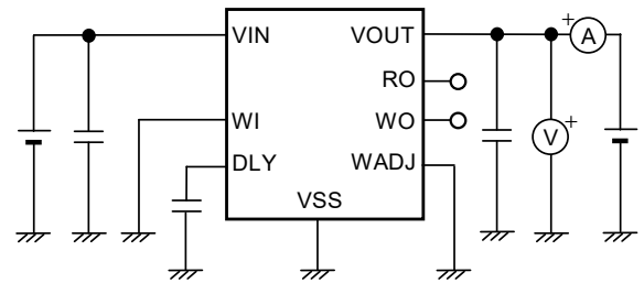
図23 測定回路2
