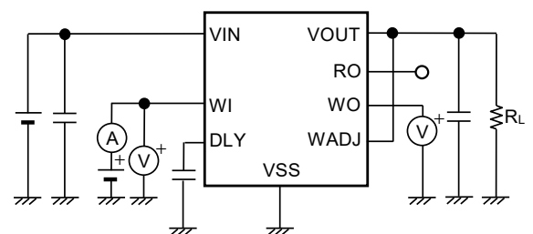
図29 測定回路8
