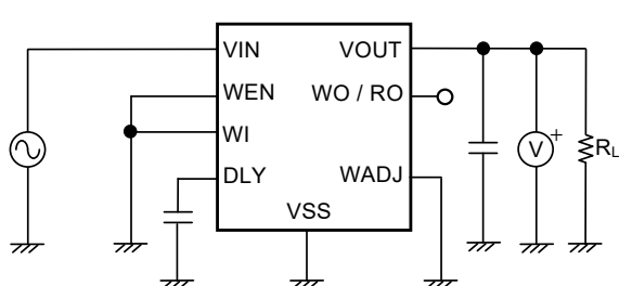
図14 測定回路3
