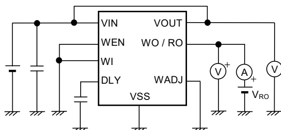
図16 測定回路5
