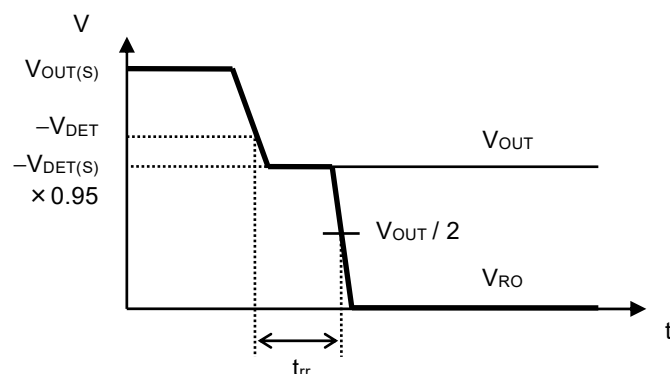
図7 リセット反応時間
