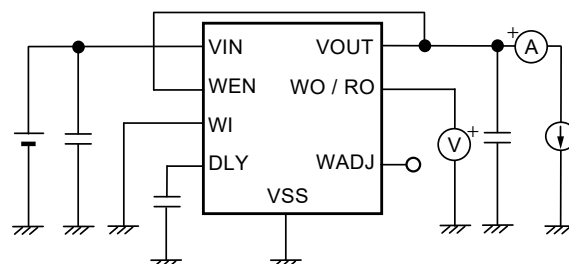
図17 測定回路6
