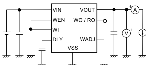
図12 測定回路1
