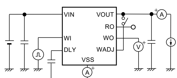
図31 測定回路10
