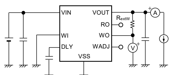
図27 測定回路6
