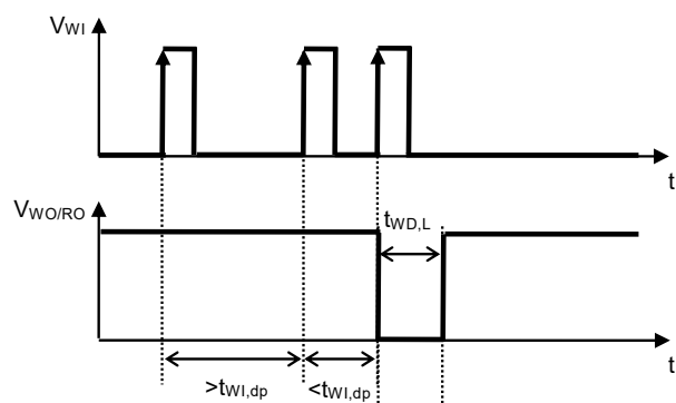
図9 ウォッチドッグダブルパルス検出時間
