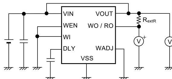
図15 測定回路4
